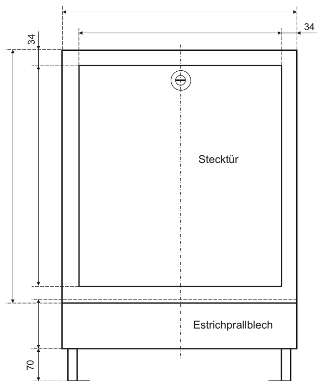
Frontansicht
